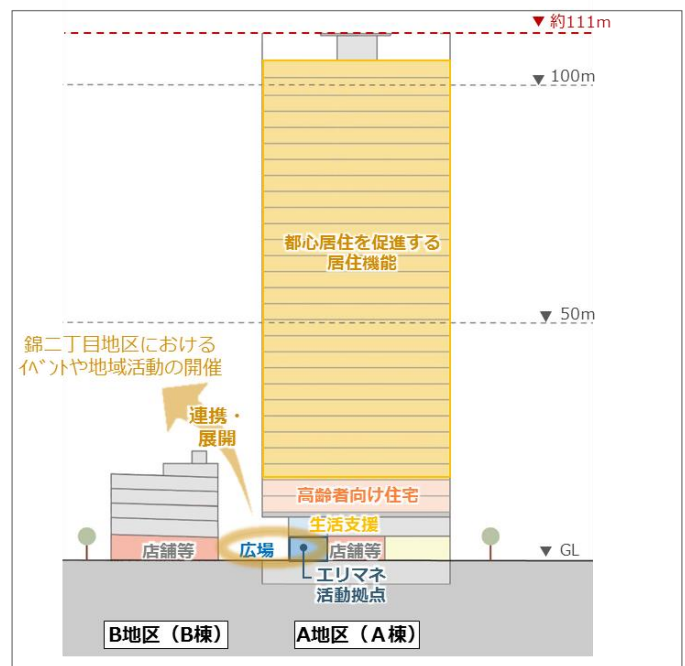
■ 断面イメージ (X 断面)
