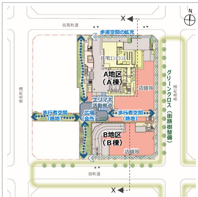
■ 1F 平面イメージ
