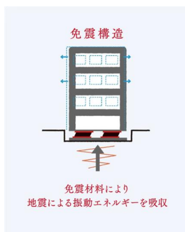
【免震構造概念図※7】
