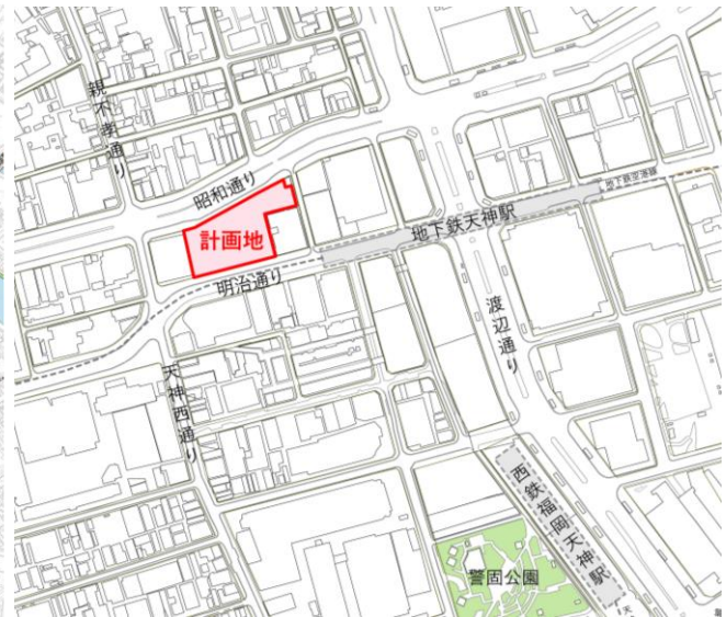
位置図
